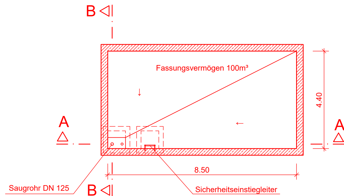
Grundriss M 1:100
