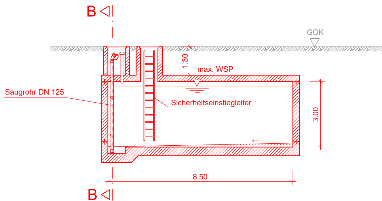
Schnitt A-A M 1:100
